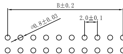
P.C.B LAYOUT
